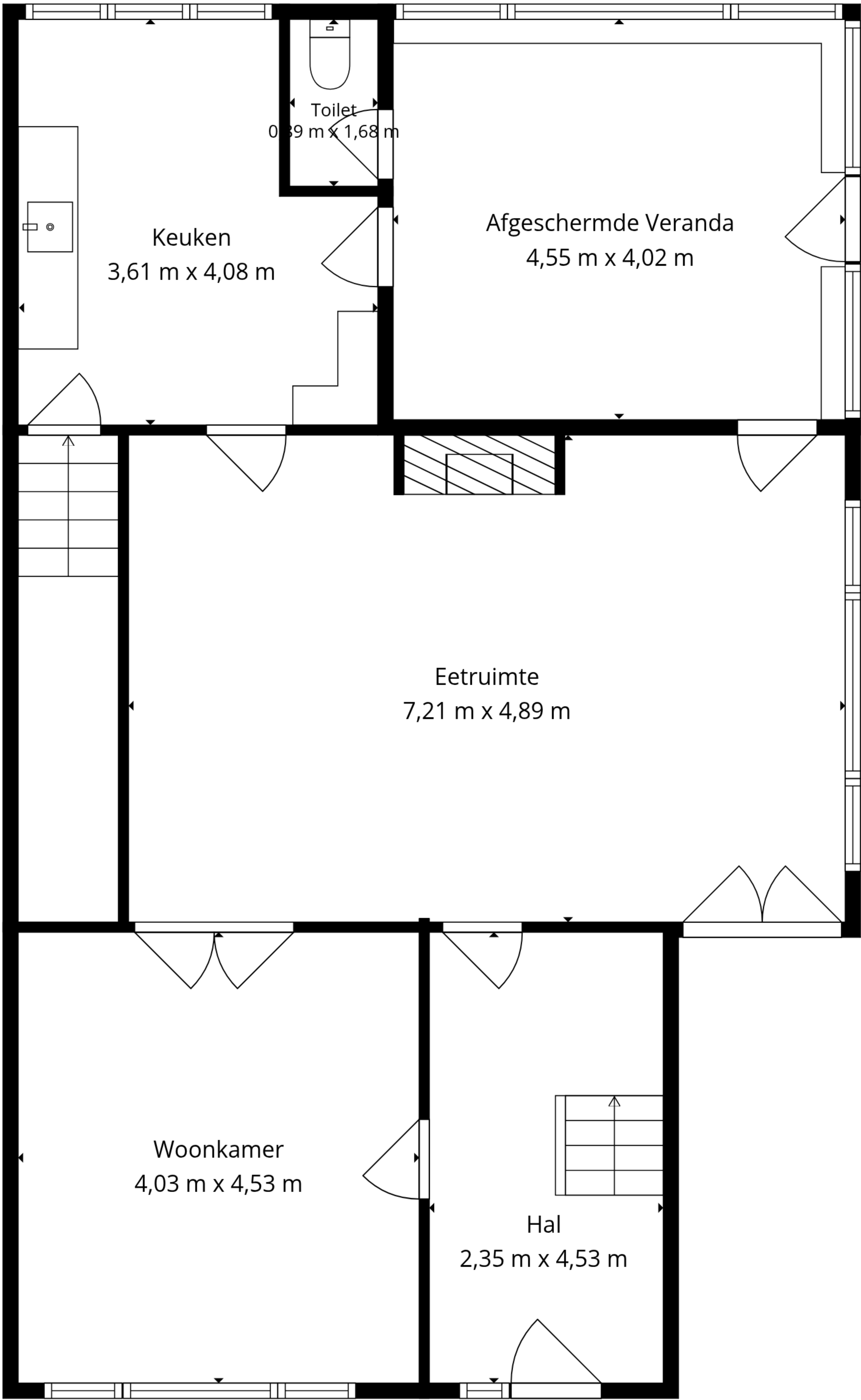
1e Verdieping
